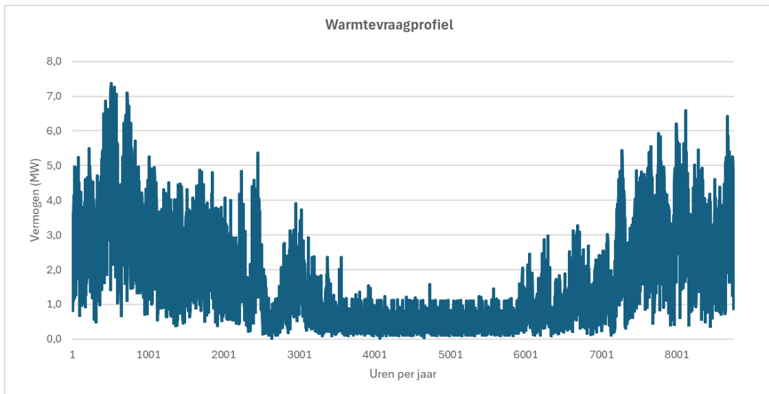
Afbeelding 3.7 Voorbeeld warmtevraagprofiel
