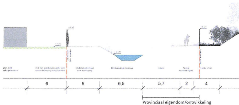
Figuur 25: Dwarsdoorsnede noordoostelijke rand plangebied
