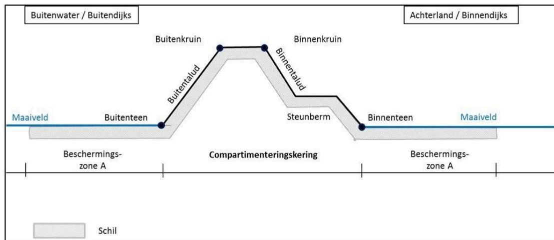
Figuur 1: ligging schil compartimenteringskering
