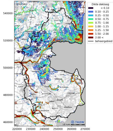
Dikte van deklaag (Veenkaart + Holoceen) in meters
