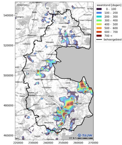
Formatie van Boxtel, eerste kleige eenheid ('BXk1')
