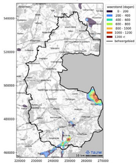
Formatie van Boxtel, tweede kleige eenheid ('BXk2')
