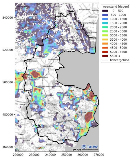
Formatie van Drenthe-Gieten, eerste kleige eenheid ('DRGk1')
