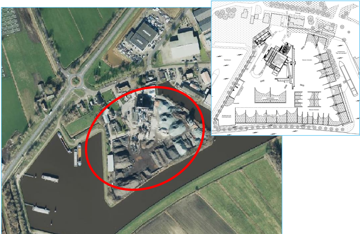
Figuur 1.1: Invulling terrein KAS
