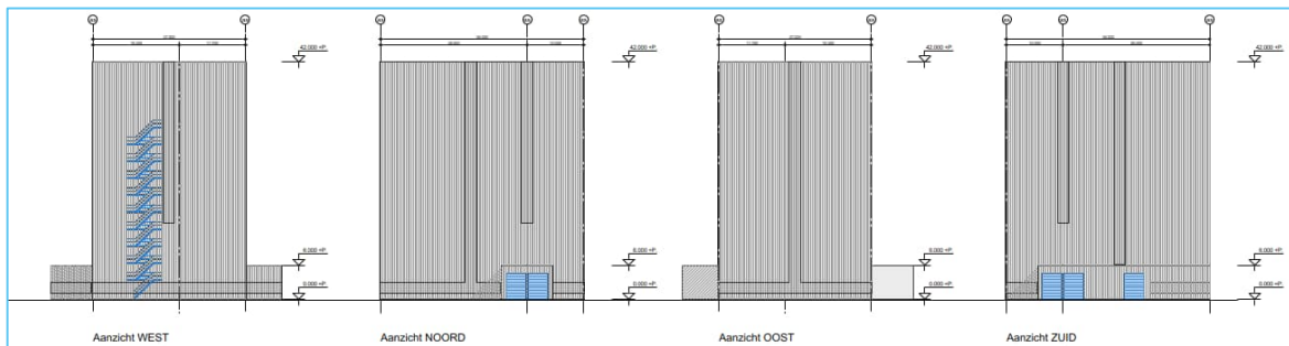
Figuur 3.2: Opbouw asfaltgebouw
