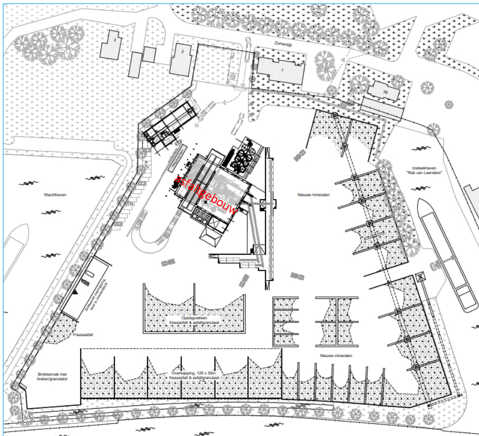
Figuur 3.1: Invulling terrein KAS
