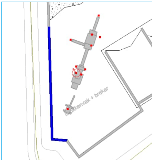
Figuur 5.1: Te verhogen deel keerwand met een afscherming van 2 meter hoog over een lengte van circa 56 meter
