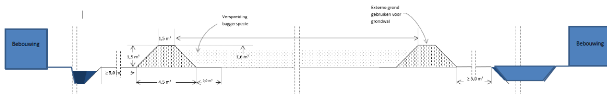
DWARSPROFIEL 1A – 1a
