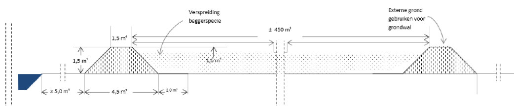
DWARSPROFIEL 2B – 2b
