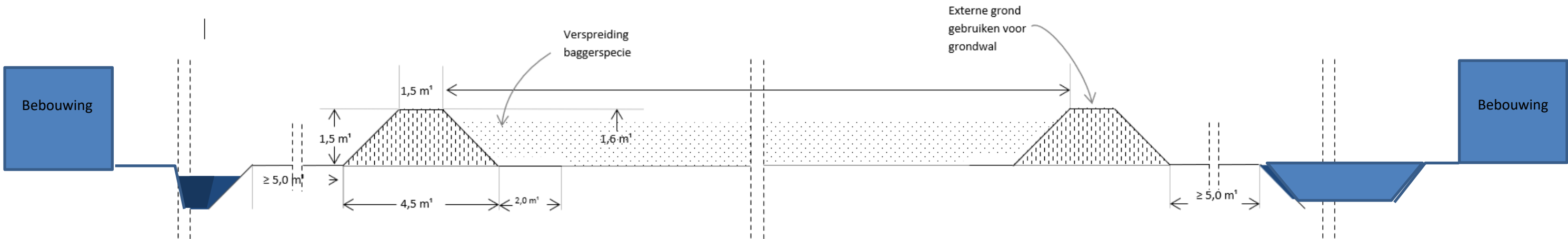
DWARSPROFIEL 1A – 1a
