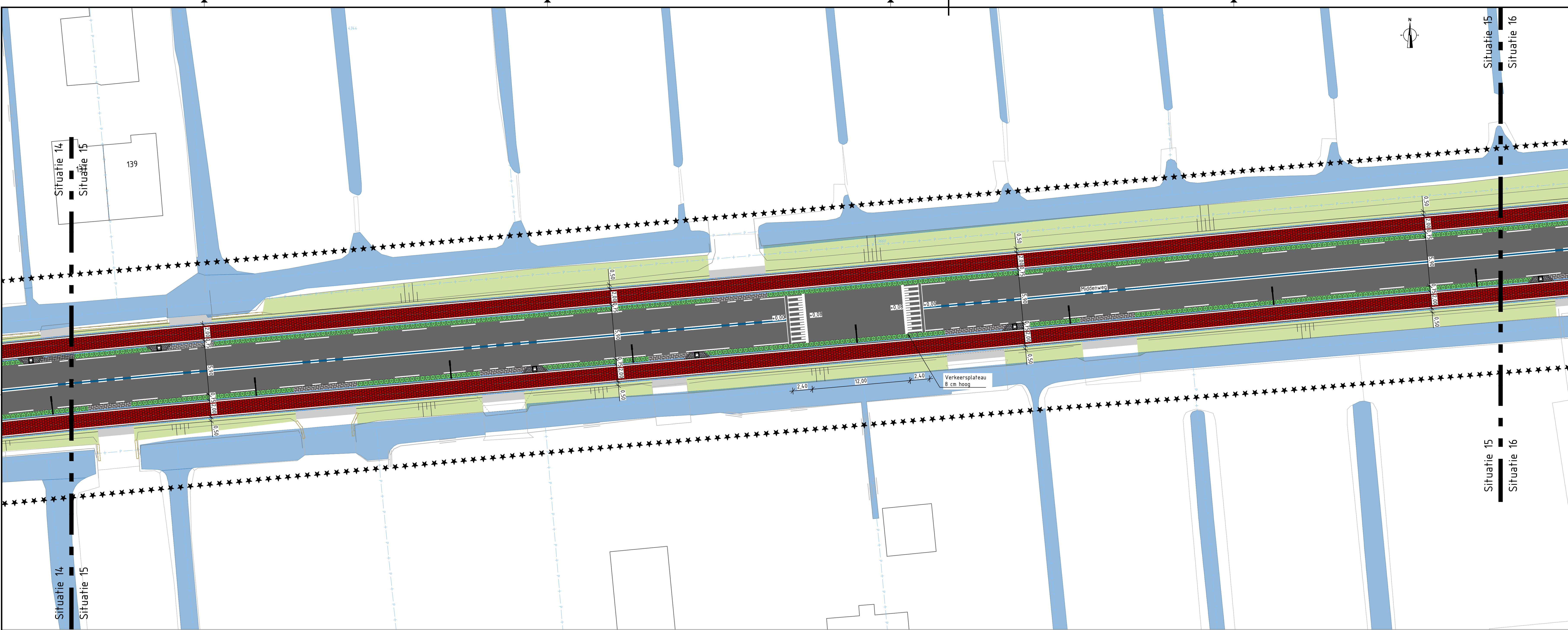
Situatie 15 SCHAAL 1:200
