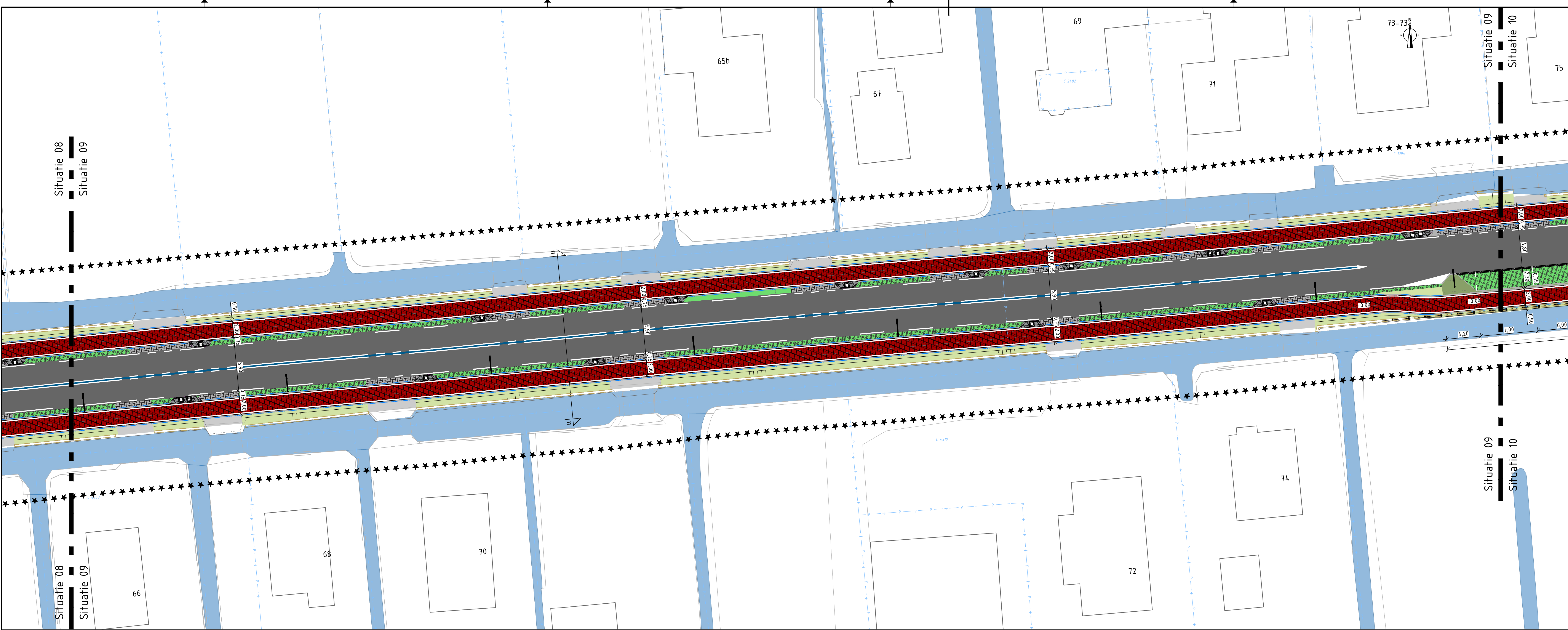
Situatie 09 SCHAAL 1 : 200
