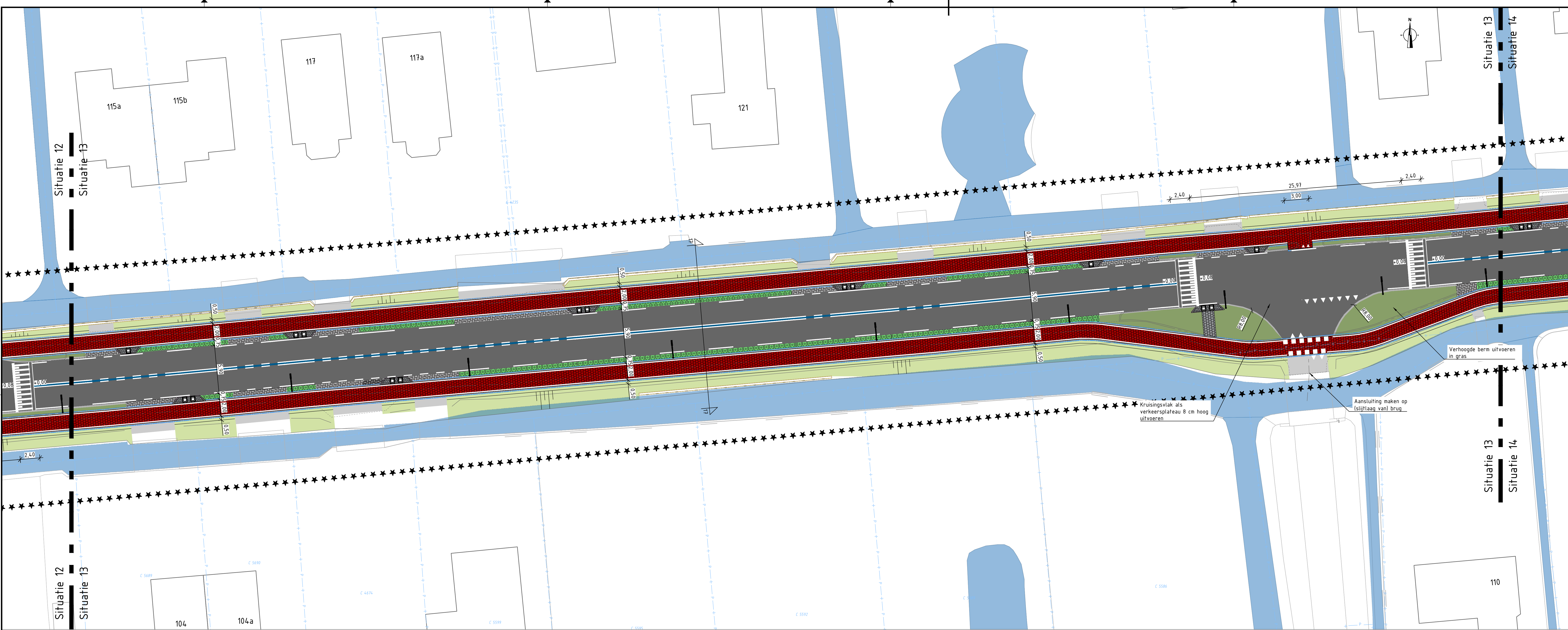
Situatie 13 SCHAAL 1 : 200
