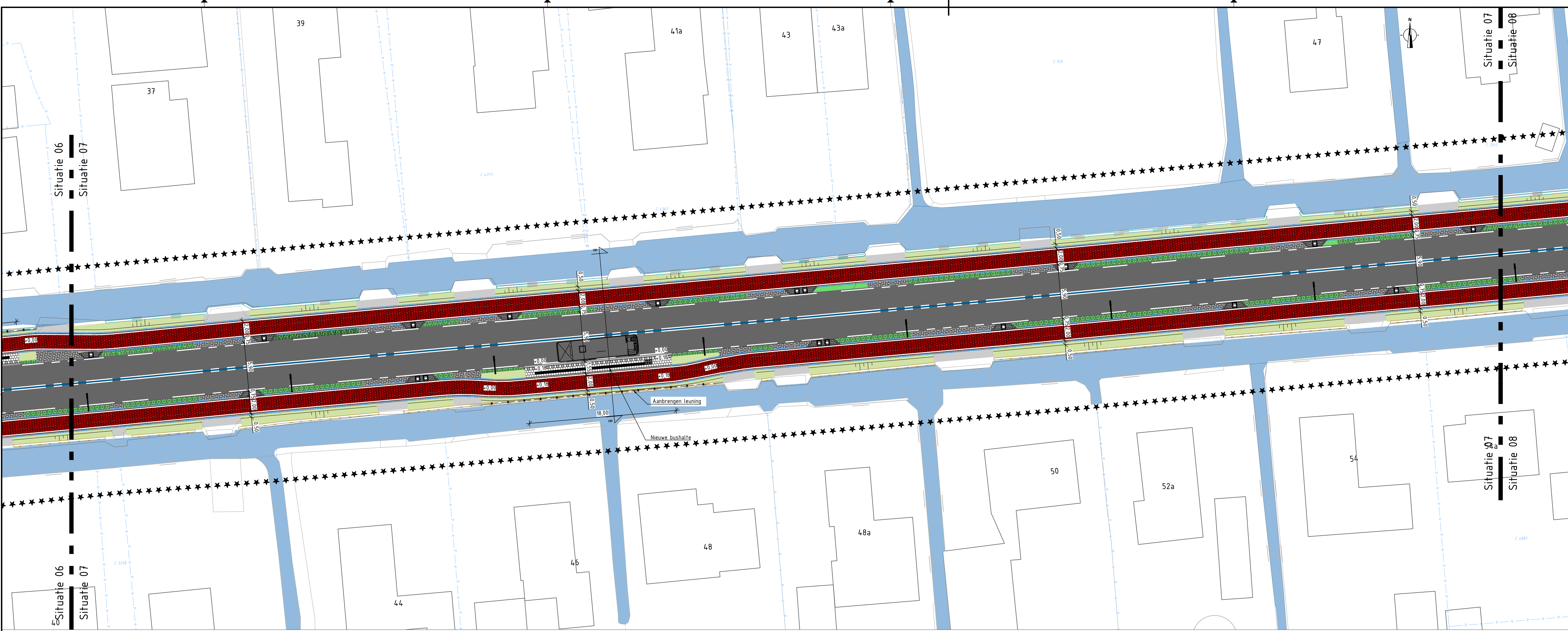
Situatie 07 SCHAAL 1 : 200
