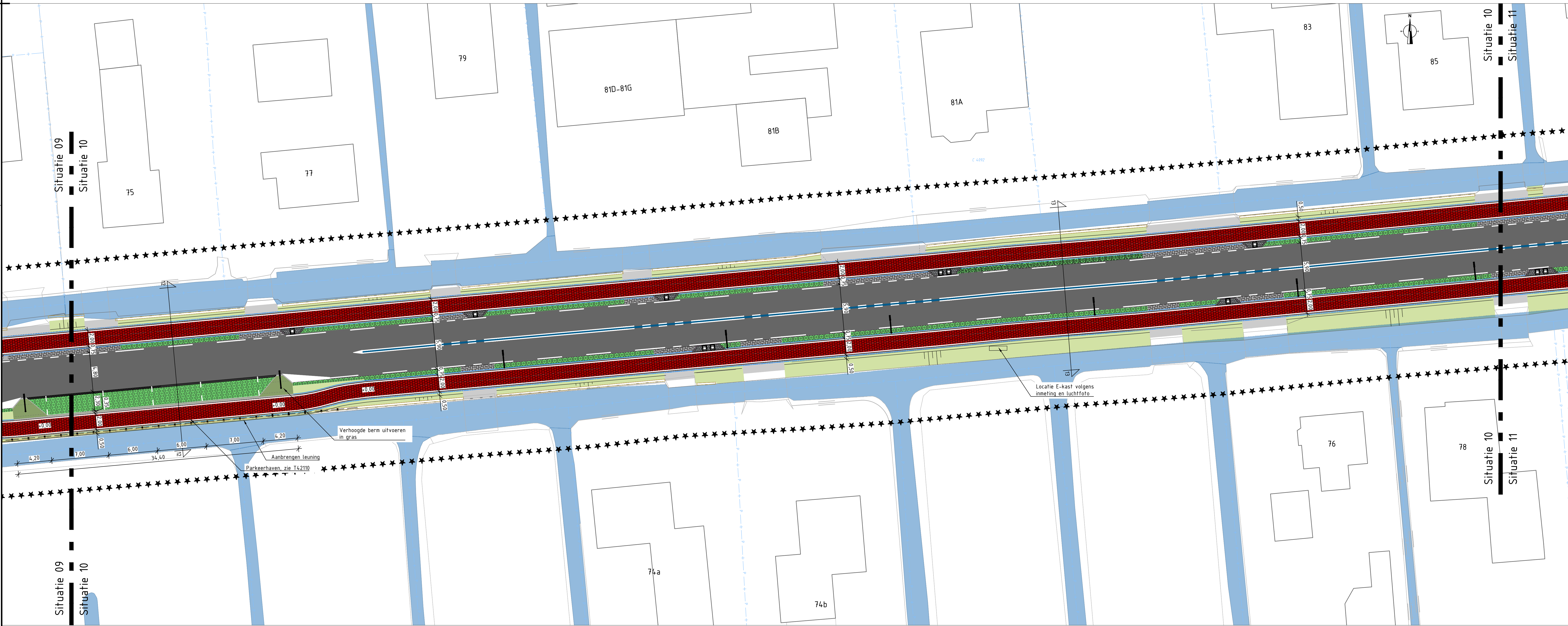
Situatie 10 SCHAAL 1 : 200
