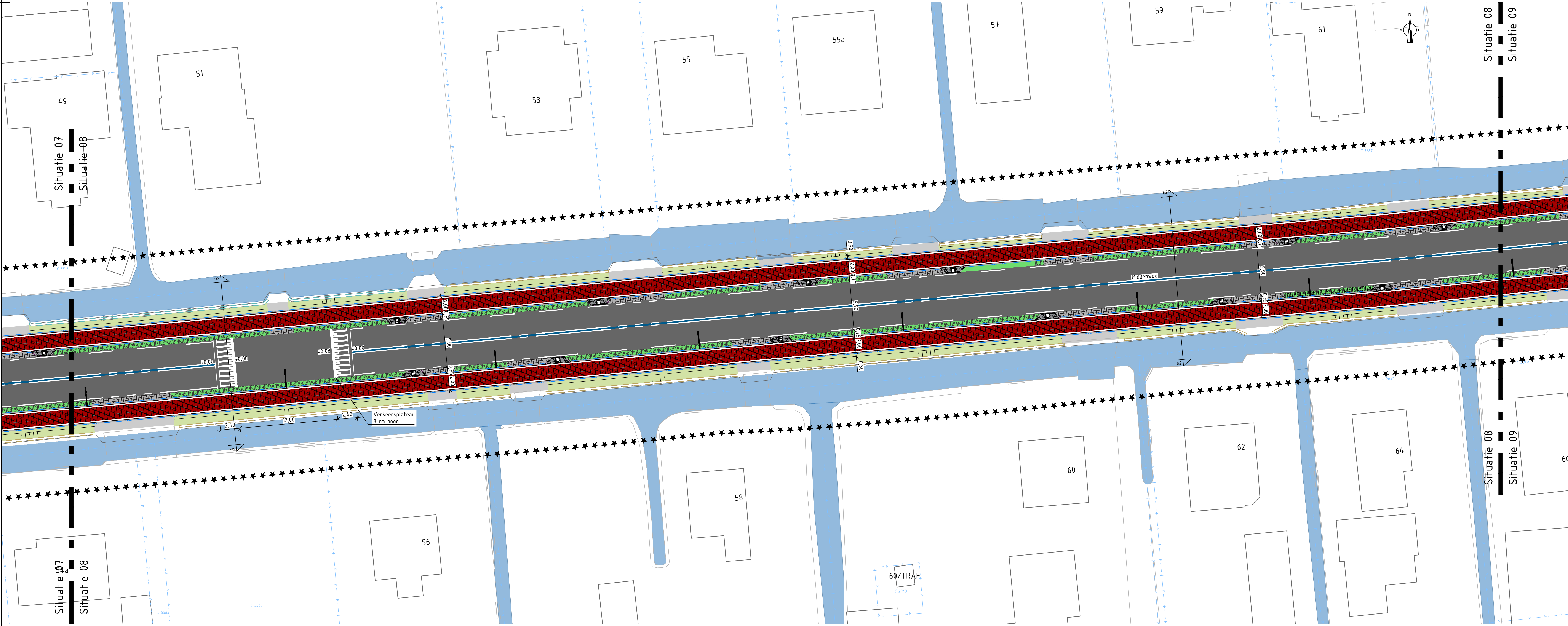
Situatie 08 SCHAAL 1 : 200
