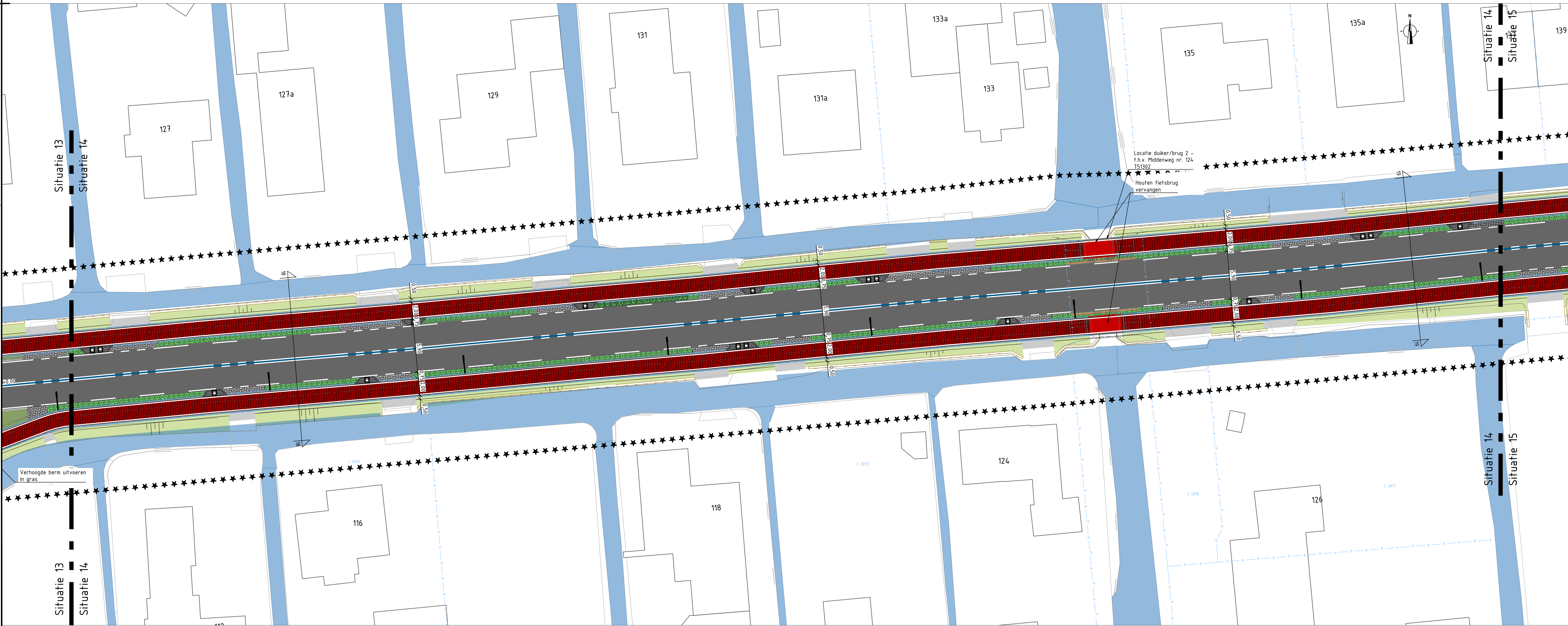
Situatie 14 SCHAAL 1 : 200
