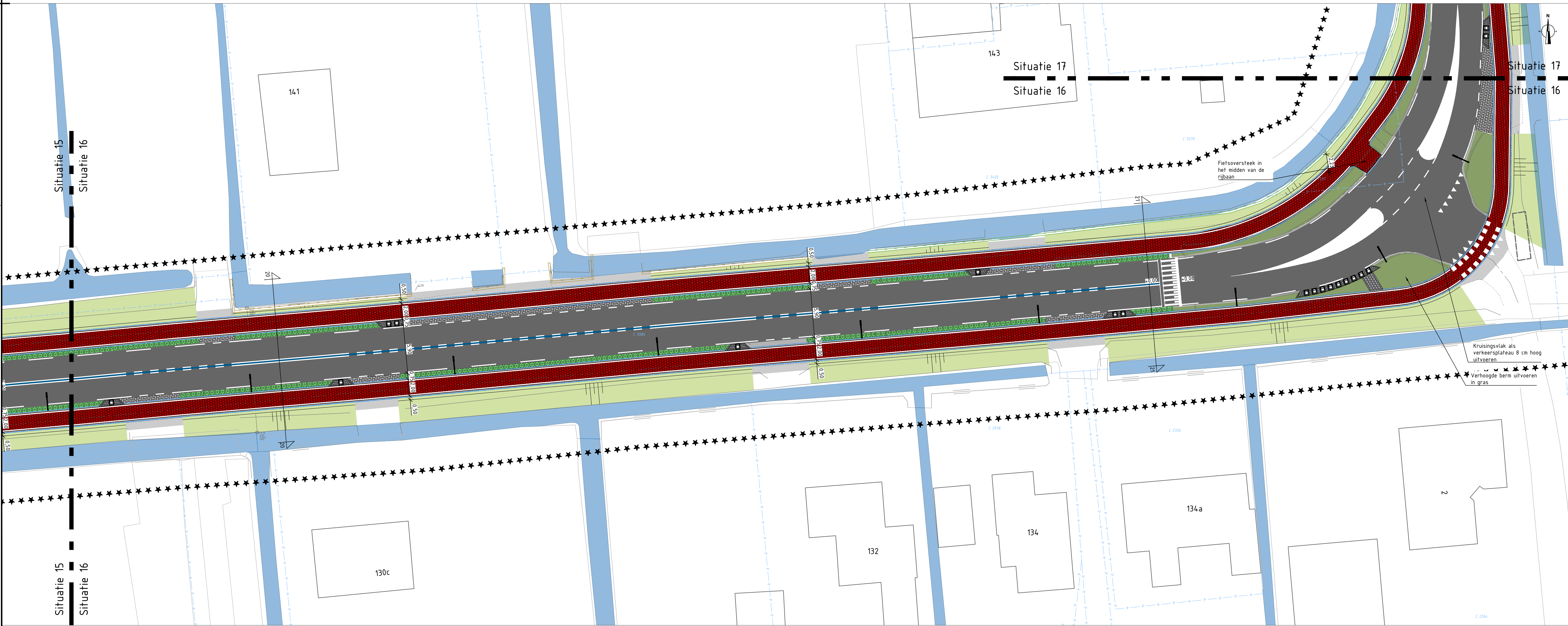
Situatie 16 SCHAAL 1:200
