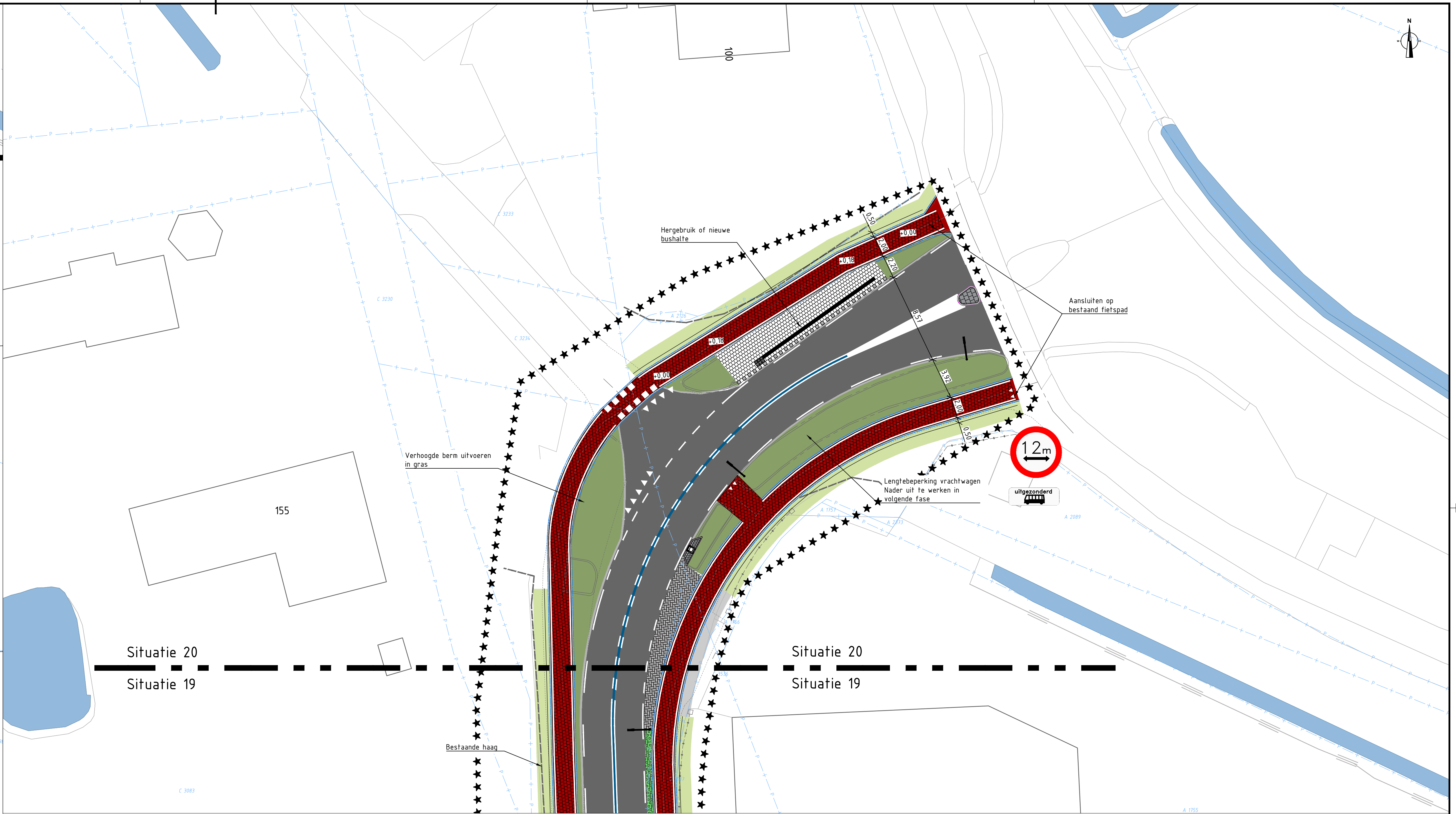
Situatie 20 SCHAAL 1 : 200
